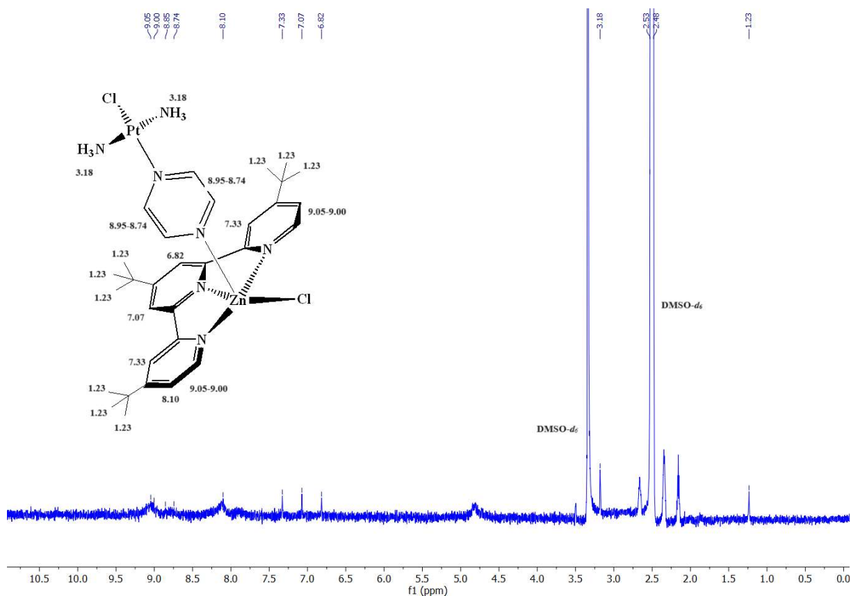
Слика 11. Спектри карактеризације \{[trans\text{-PtCl}(\text{NH}_3)_2(\mu\text{-пиразин})\text{ZnCl}(\text{terpy}^{t\text{Bu}})](\text{ClO}_4)_2\} комплекса
