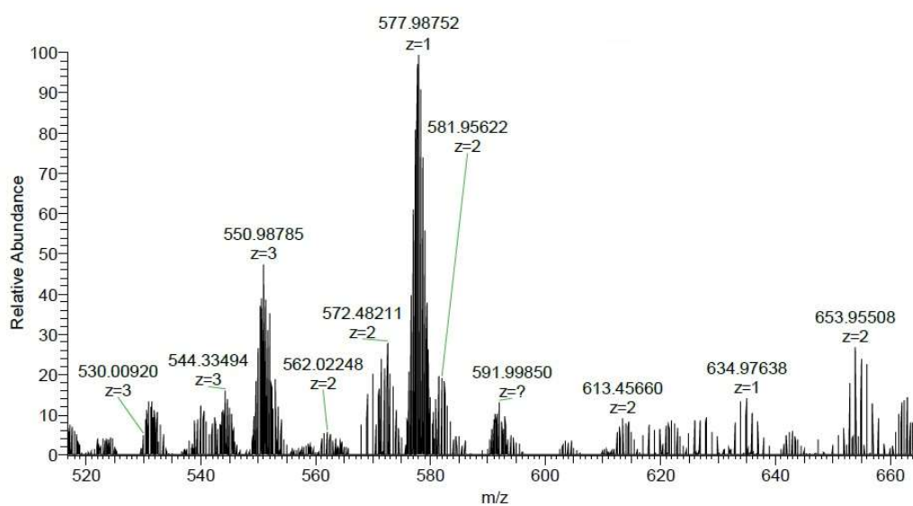
Слика 9. Спектри карактеризације [\text{ZnCl}_2(\text{terpy}^{\text{Bu}})] комплекса
