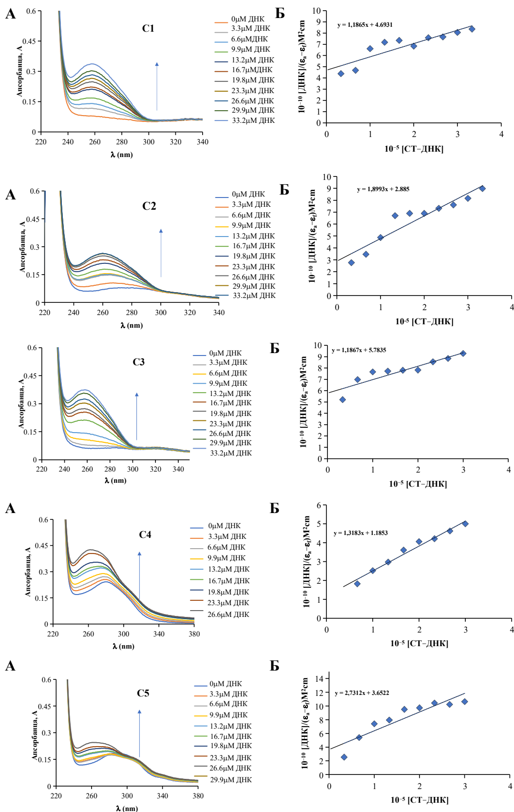
Слика 19. (А) Апсорпциони спектри C1-C5 комплекса у присуству растућих концентрација СТ-ДНК различитих концентрација. Пораст апсорпције означен је стрелицом. (Б) Зависност [\text{CT-ДНК}]/(\epsilon_A - \epsilon_F) = y у функцији [\text{CT-ДНК}] .
