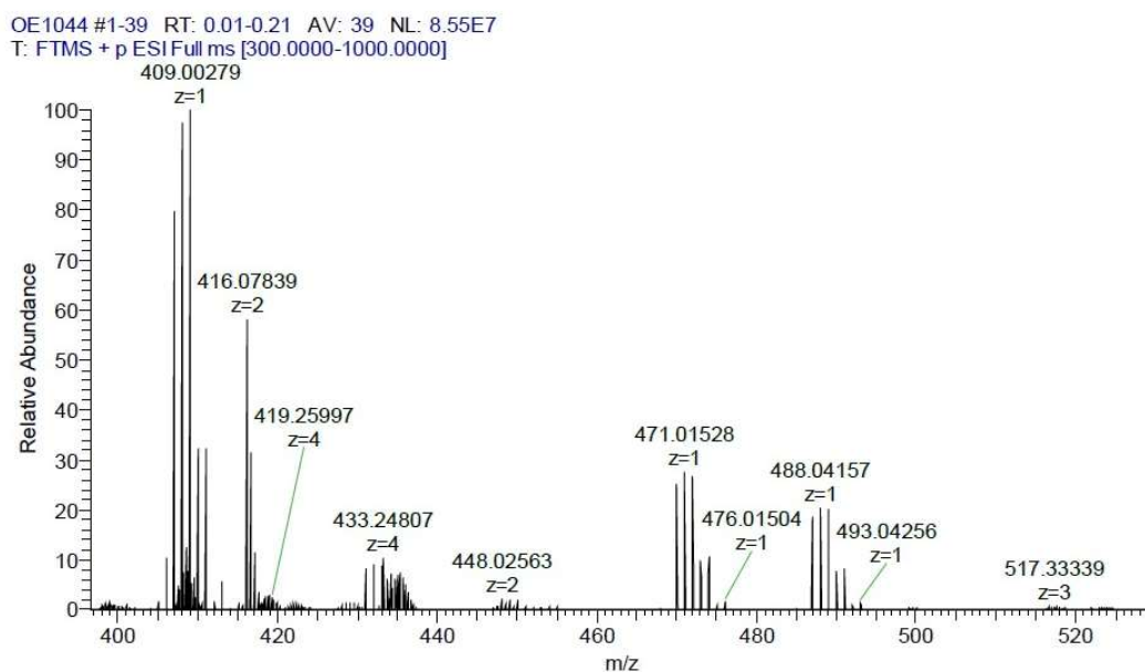
Слика 10. Спектри карактеризације
